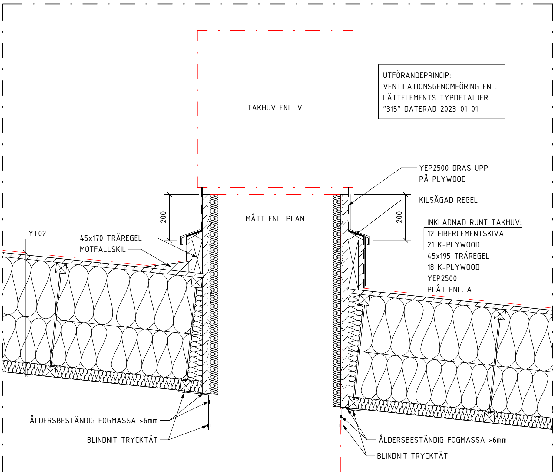
B - B 1 : 10
