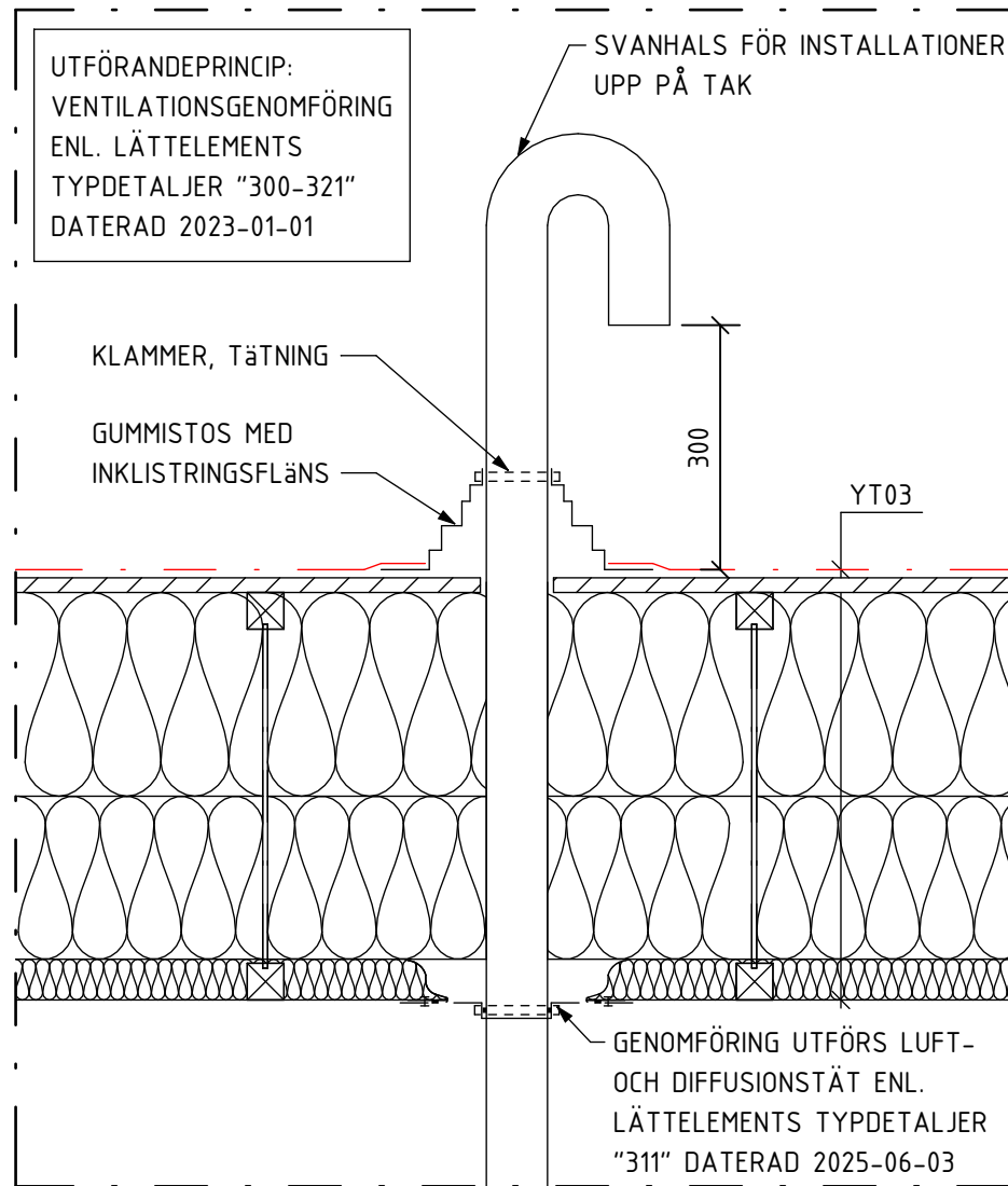
PRINCIPDETALJ 1:10
