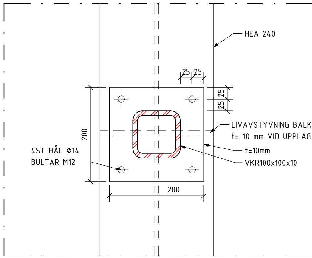
a - a 1 : 5
