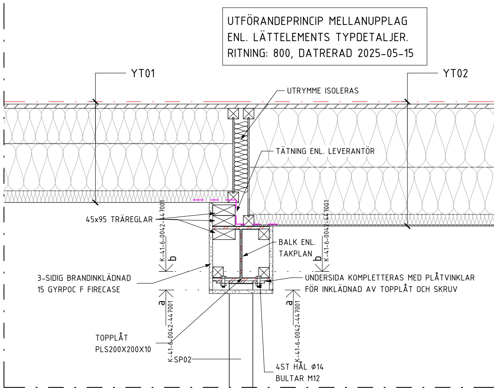
A - A 1 : 10
