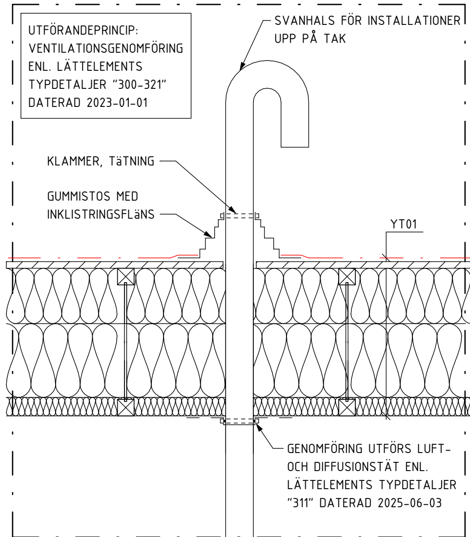
PRINCIPDETALJ 1:10
